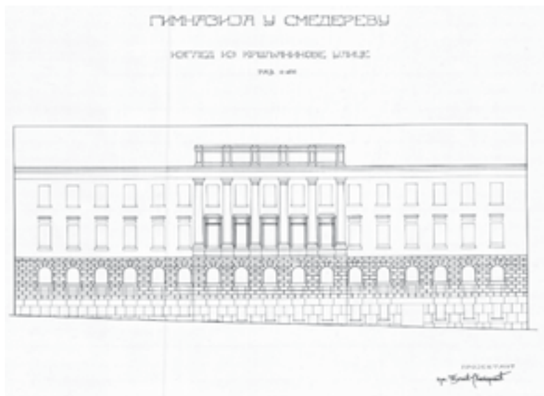
|Сл. 6. Арх. Јованка Бончић Катеринић, Пројекат Гимназије у Смедереву, изглед из Кршљанинове улице Извор: АЈ, МГ, VII- 051- Гимназија у Смедереву II/3
